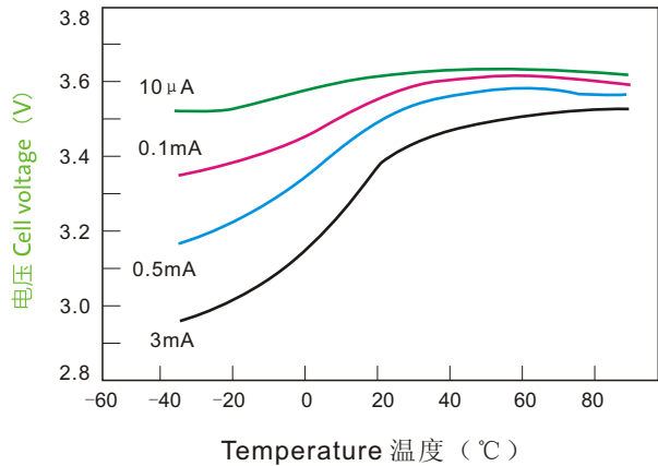
Discharge characteristic 放电特性 (25°C)
