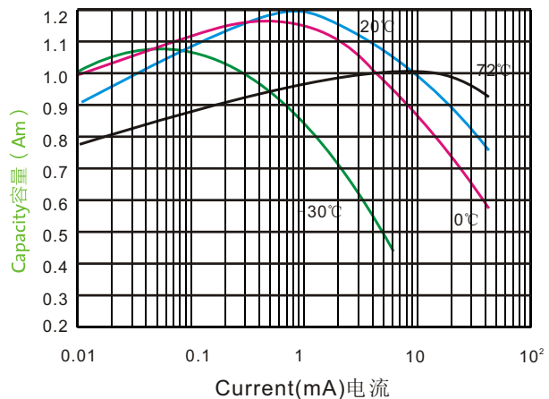
Capacity vs current 容量vs电流
