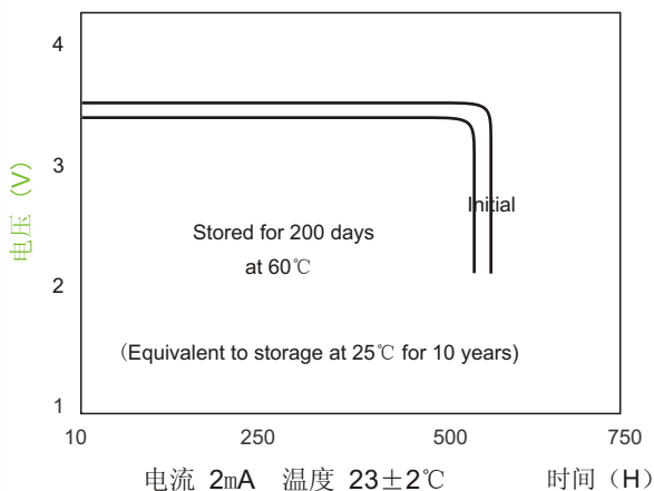
Storage characteristics 存储特性
